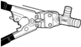
将卡箍套上管路并用工具闭合卡箍耳朵部位, 直至卡箍完全被卡紧后工具才可释放。
