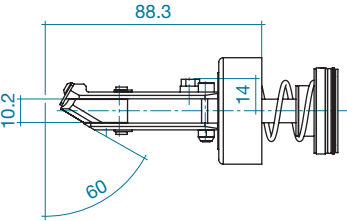
钳爪倾角 60°
