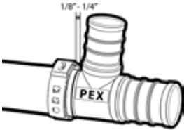
“卡箍”与“管路末端”之间建议相距1/8"- 1/4"。
