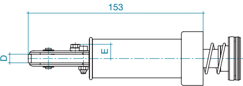
延伸 80 mm
