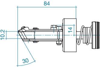
钳爪倾角 30°
