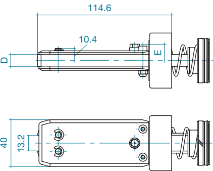
延伸 42 mm, 窄
