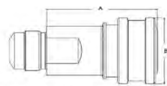
图 1: 阴接头部分
