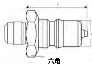
图 2: 阳接头部分
