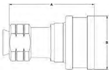
图 1: 阴接头部分
