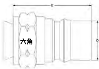
图 2: 阳接头部分
